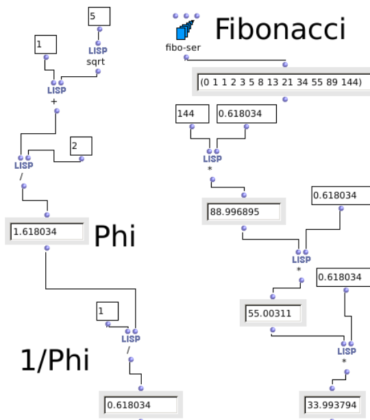
Figura 16 – A fórmula para encontrar a constante 1/\Phi e sua relação com a série de Fibonacci, testada no OpenMusic.
