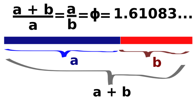
Figura 15 – Razão geométrica da proporção áurea
