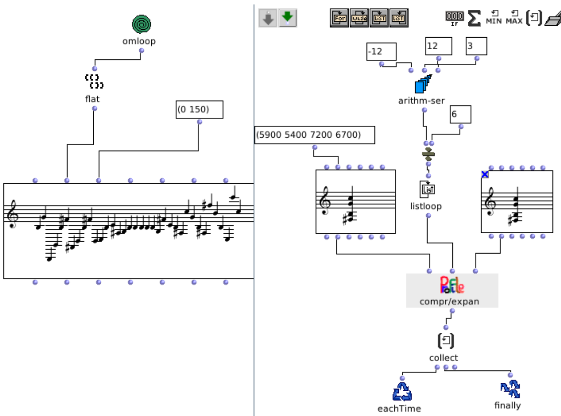
Figura 75 – Comprime e expande em passos de 3 intervalos simétricos, abrindo e fechando os acordes baseados em uma célula Z.
