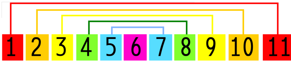
Figura 79 – Equivalência de intervalos por inversão
