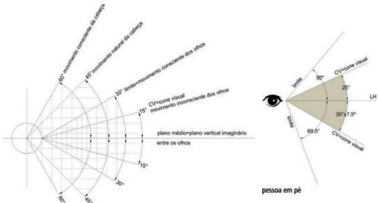
Figura 4 – Diagrama do olho humano e cones visuais
