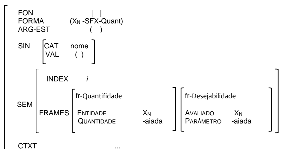
Figura 8 – Matriz atributo valor para a CQMS genérica
