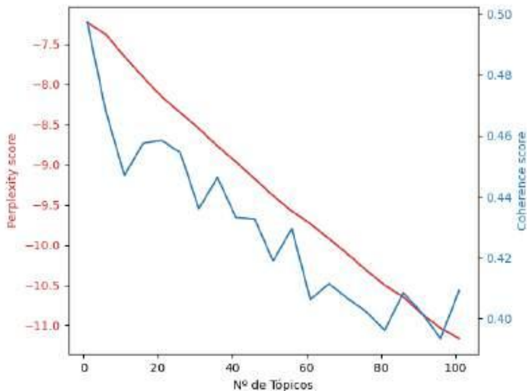
Figura 12 - Gráfico dos valores de coerência e perplexidade para cada número de tópicos testado
