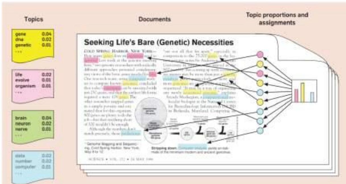
Figura 11 - Modelagem de tópicos por meio de técnica LDA
