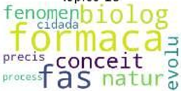
Tópico 18
