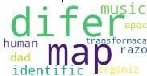
Tópico 13
