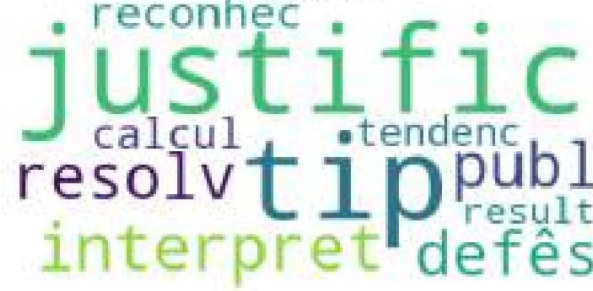
Tópico 15
