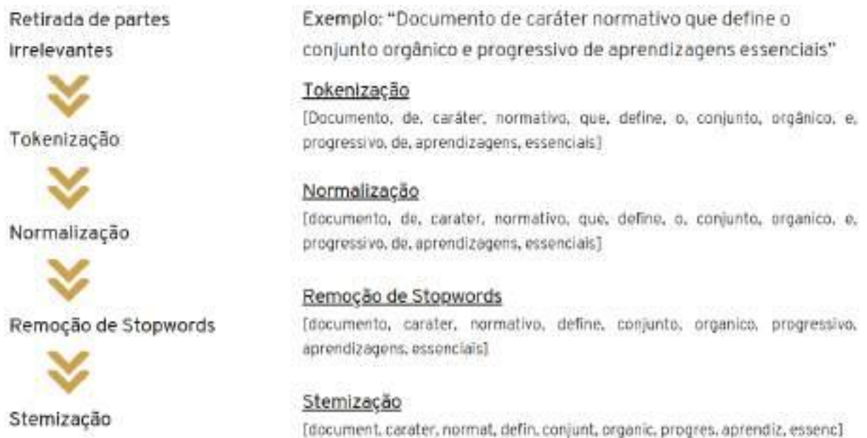
Figura 9 - Exemplo de tratamento dos dados textuais
