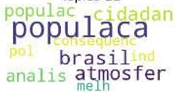
Tópico 12
