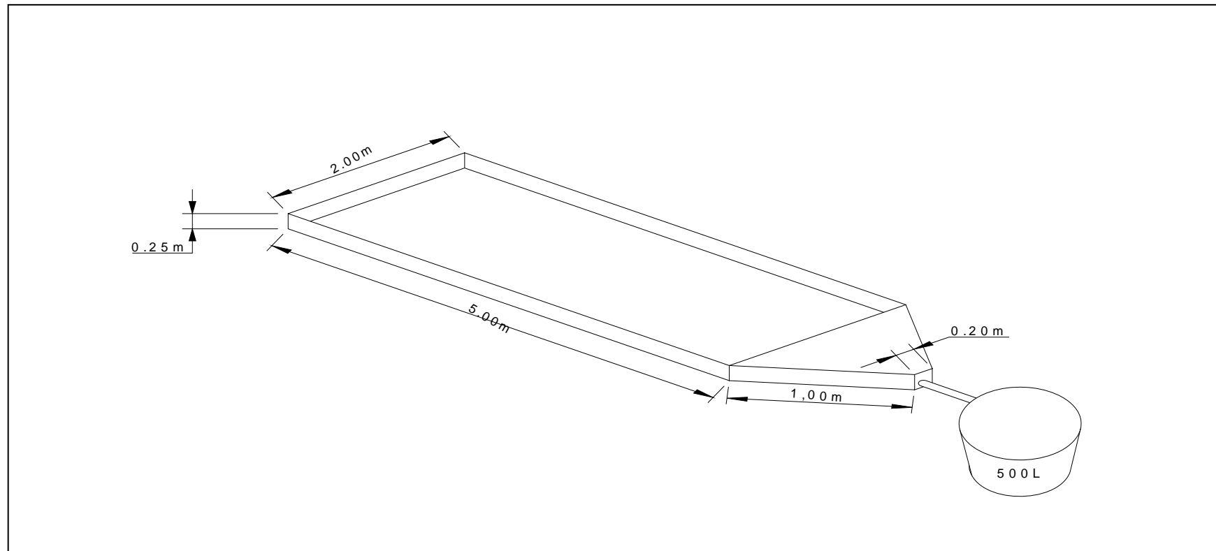
Parcela experimental de 2 x 5m, instalada no sentido do declive para aplicação de estudos de perda de solo e água.
