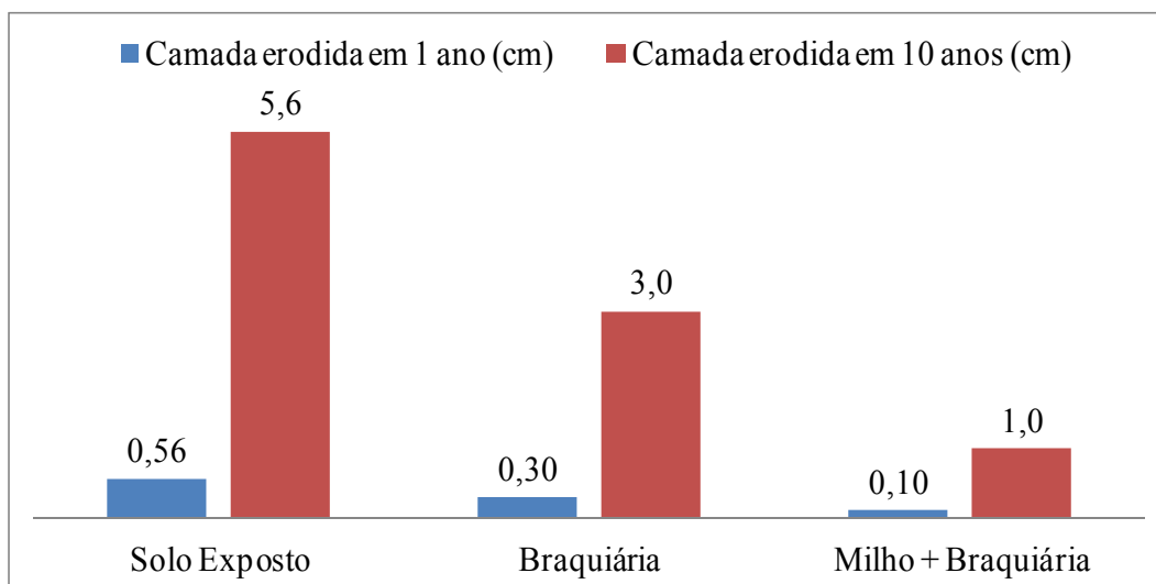
Figura 6. Perdas de solo por profundidade da camada. Para a estimativa de 10 anos foi considerada uma avaliação constante e linear, baseada na perda medida em 12 meses.
