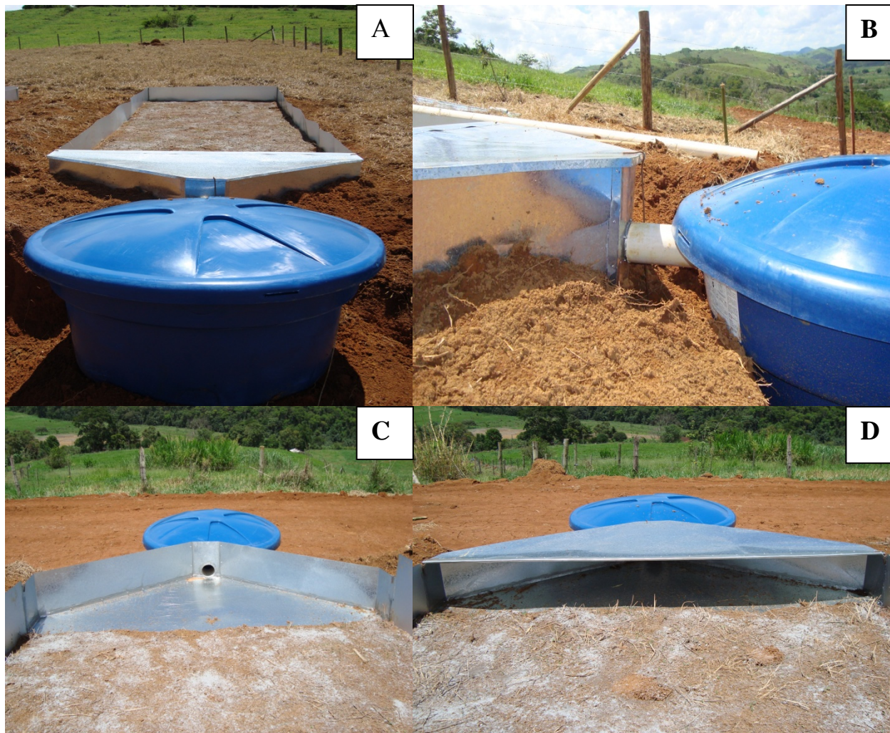
Estruturas das parcelas experimentais. Autor: CARVALHO, A. C. B.
